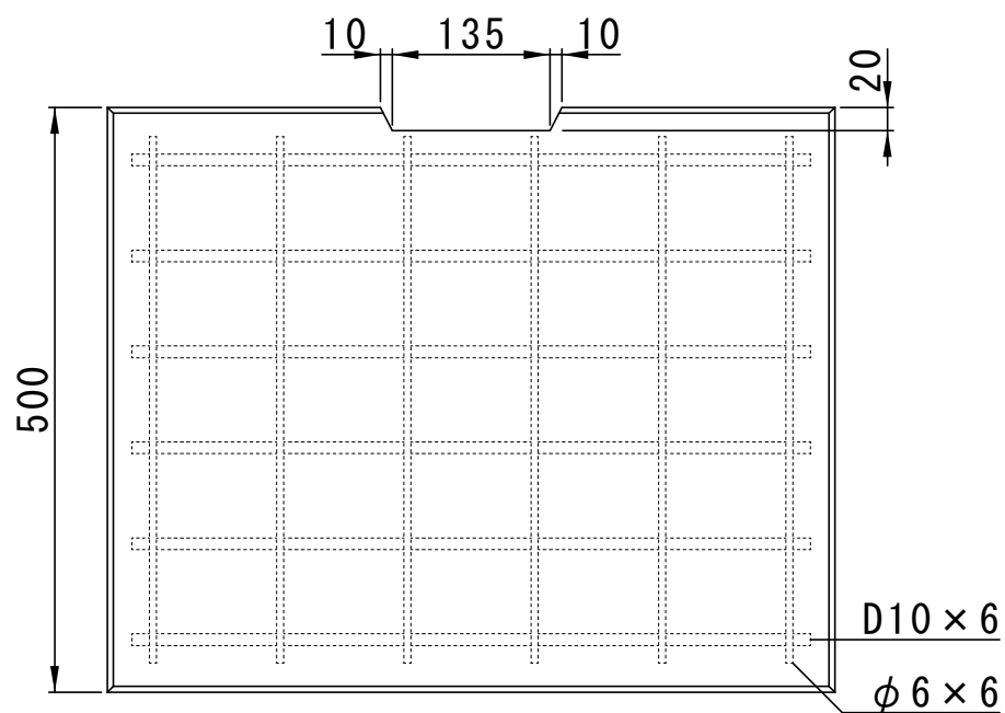
平面図
