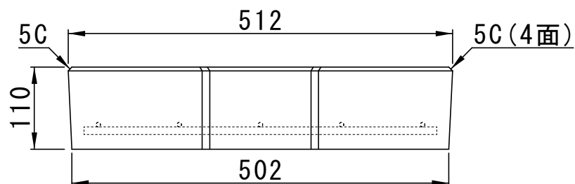
正面図
