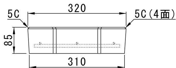
正面図
