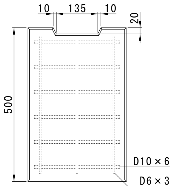
平面図
