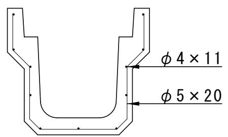
配筋図
