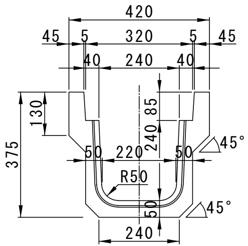
正面図
