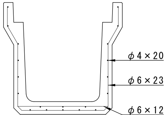
配筋図
