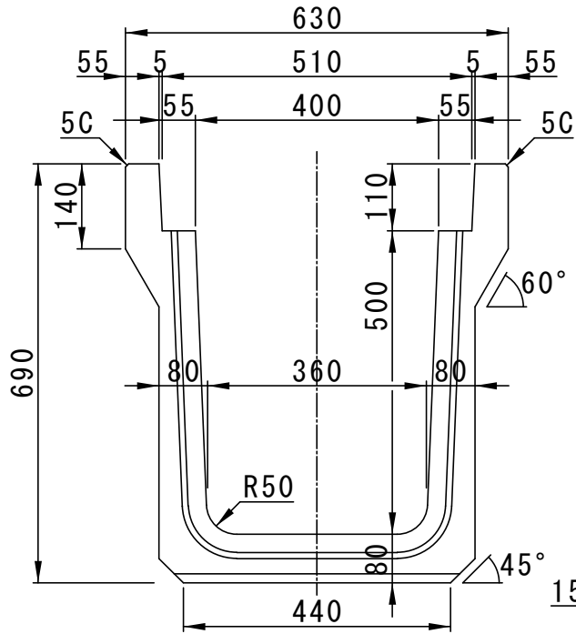
配筋図
