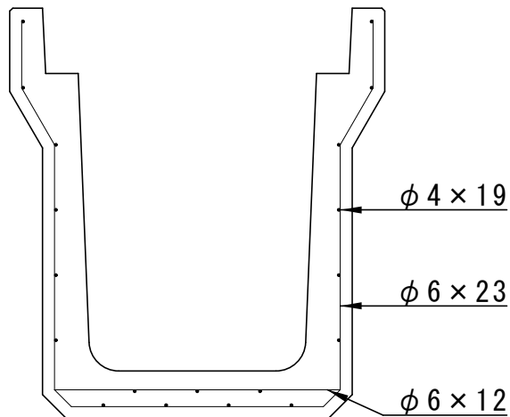
配筋図
