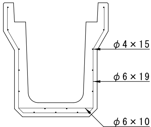
配筋図
