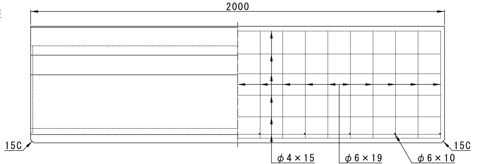
側面図
