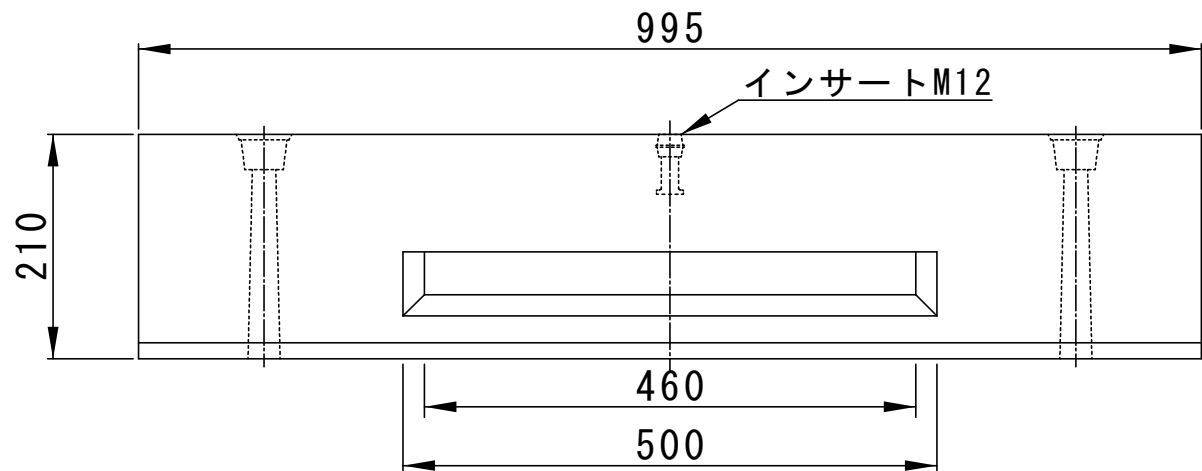
側面図
