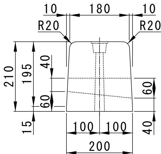
正面図
