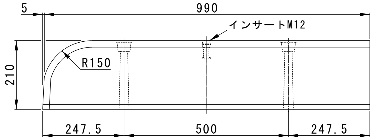
側面図
