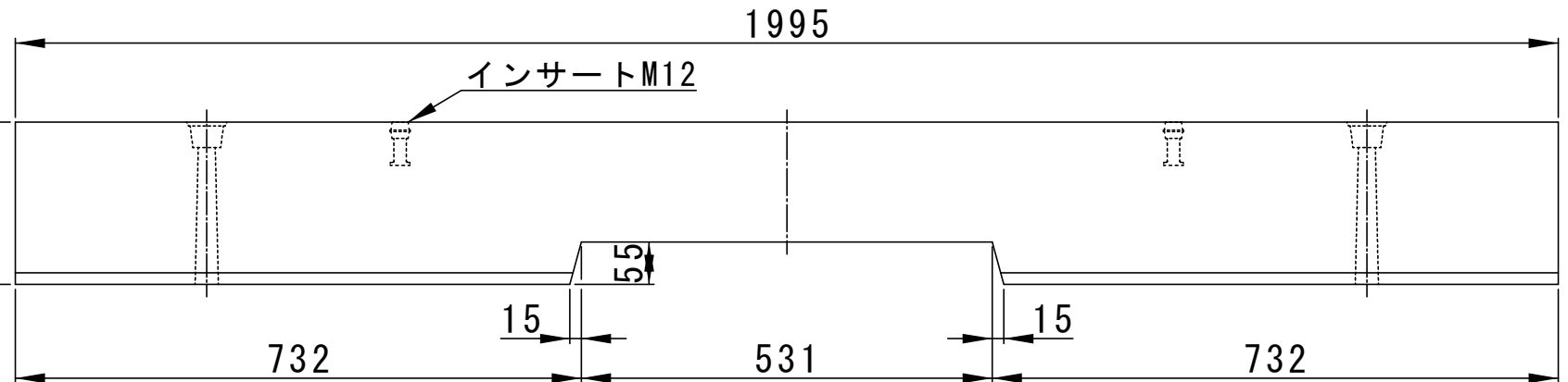
側面図
