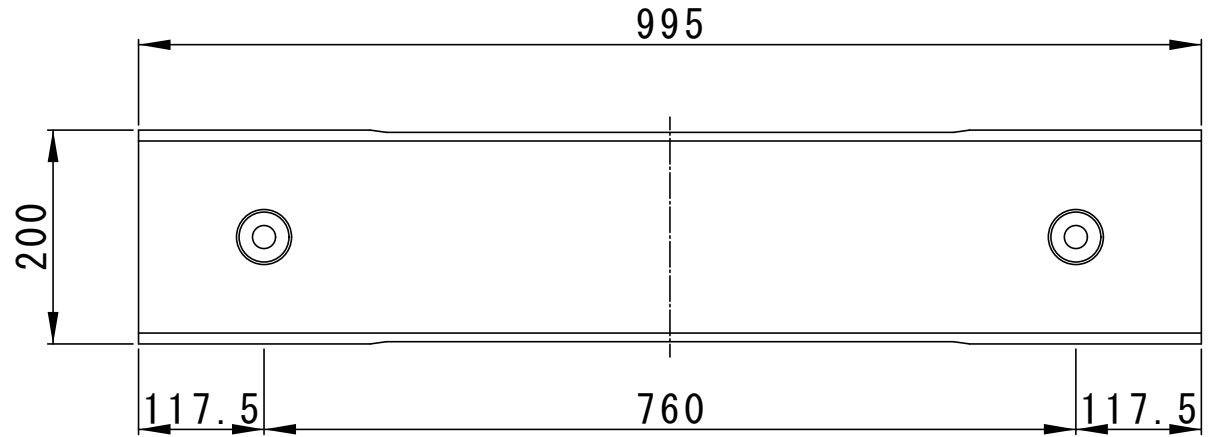
平面図
