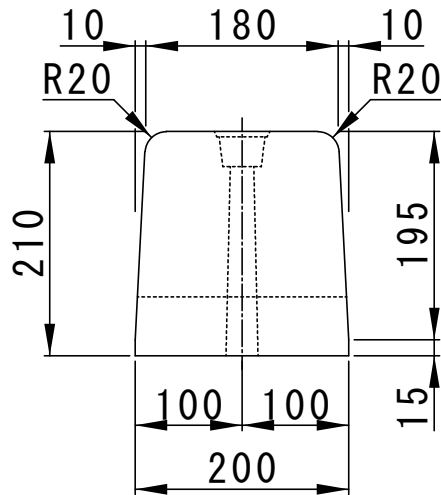
正面図
