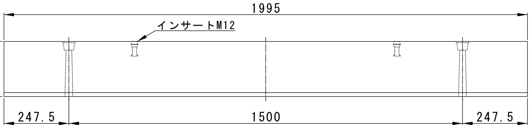
側面図
