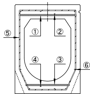
配筋図
