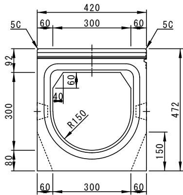
正面図
