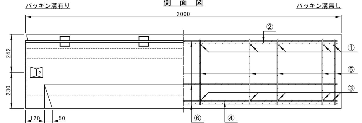
側面図
