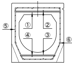
配筋図
