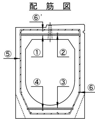
配筋図
